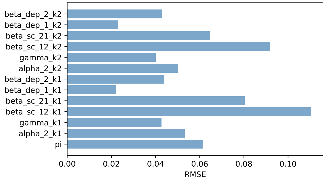
RMSE pr. parameter
