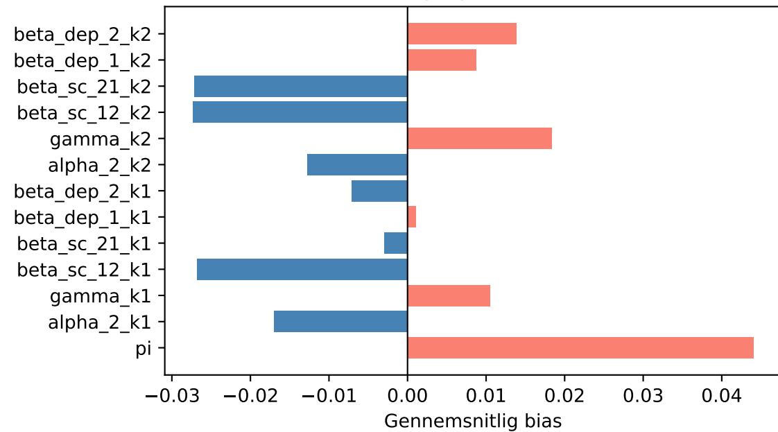
Bias pr. parameter
